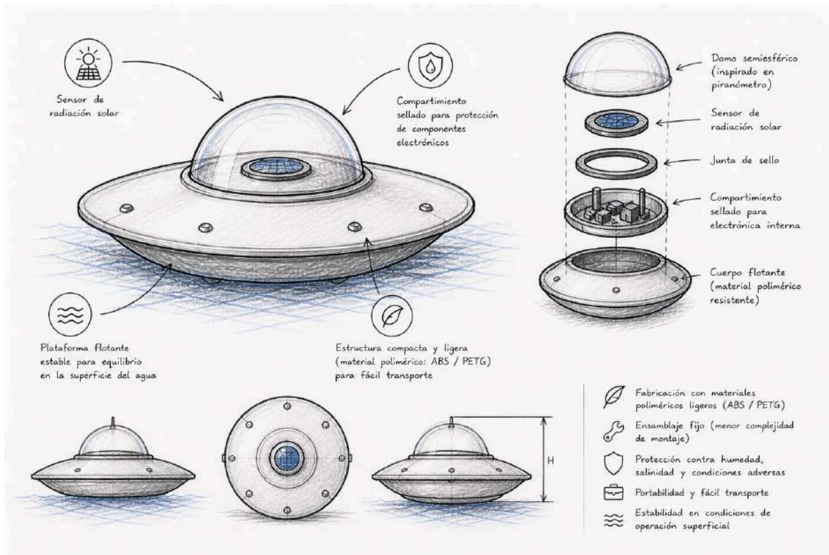
Figura 10: solución Mecánica 1
