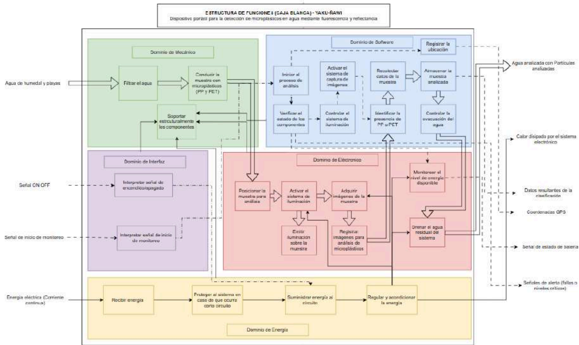
Figura 6: Estructura de funciones de YAKU-ÑAWI.
