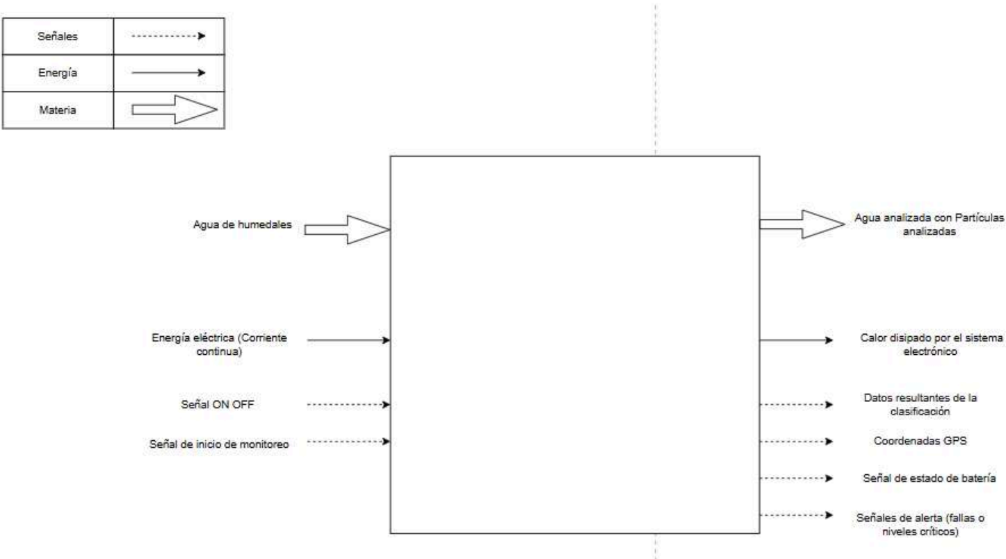
Figura 4: Caja Negra de YAKU-ÑAWI.
