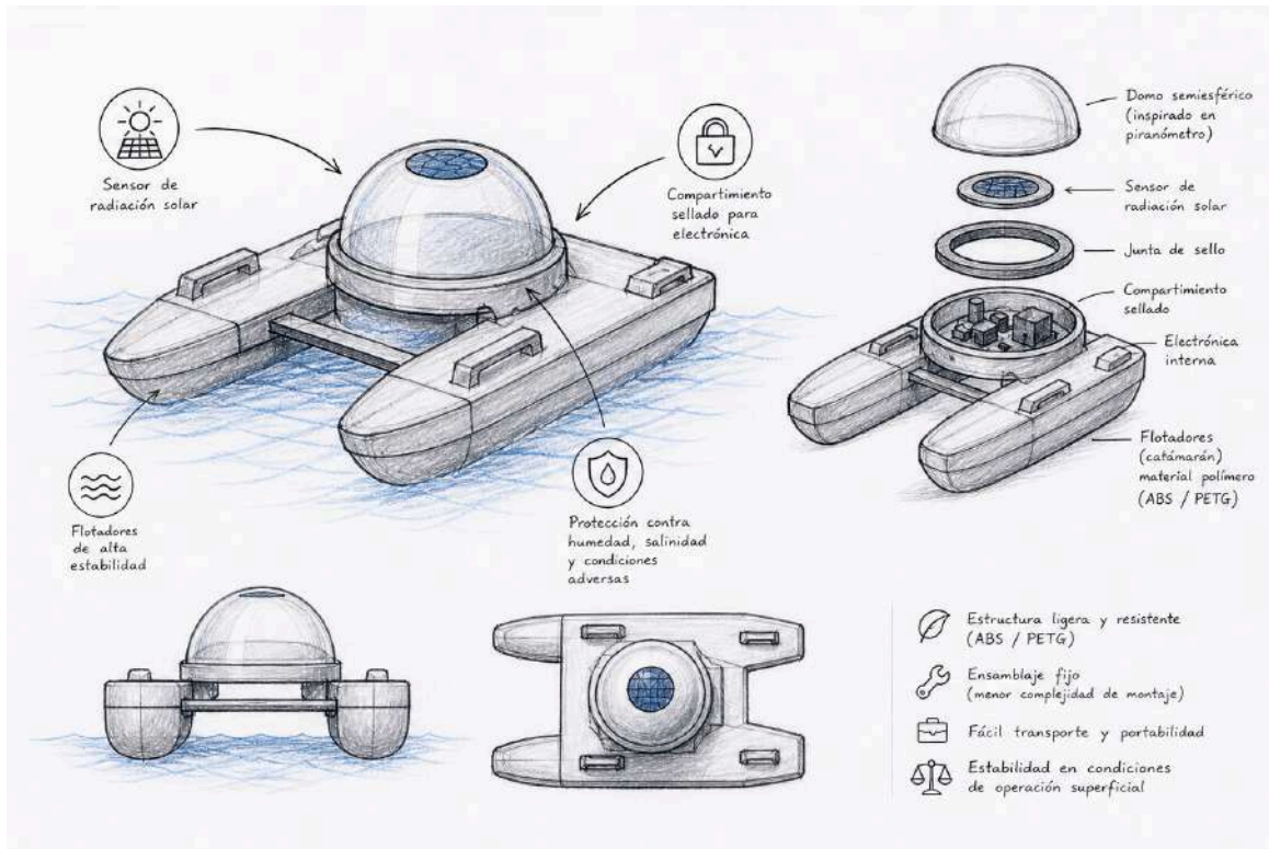
Figura 11: solución Mecánica 2
